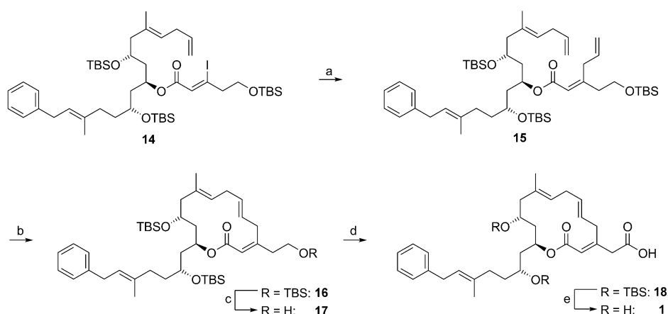
Scheme 5. a) \text{Bu}_3\text{SnCH}_2\text{CH}=\text{CH}_2 , \text{AsPh}_3 , [\text{Pd}_2(\text{dba})_3] (15 mol %), DMF, RT, 16 h, 86 %; b) Grubbs I (12 mol %), \text{CH}_2\text{Cl}_2 , RT, 3.5 h, then DMSO, RT, 17 h, 77 %; c) HF-py, pyridine, THF, 0^{\circ}\text{C} , 4 h, 81 %; d) DMP, THF, RT, 30 min, then \text{NaClO}_2 , \text{NaH}_2\text{PO}_4 \cdot \text{H}_2\text{O} , \text{tBuOH} , \text{H}_2\text{O} , 2-methyl-2-butene, RT, 20 min, 81 %; e) 5 % aq. HF in \text{CH}_3\text{CN} , 0^{\circ}\text{C} , 3 h, 88 %. DMP = Dess–Martin periodinane, Grubbs I = bis(tricyclohexylphosphine)benzylidene ruthenium(IV)dichloride.
